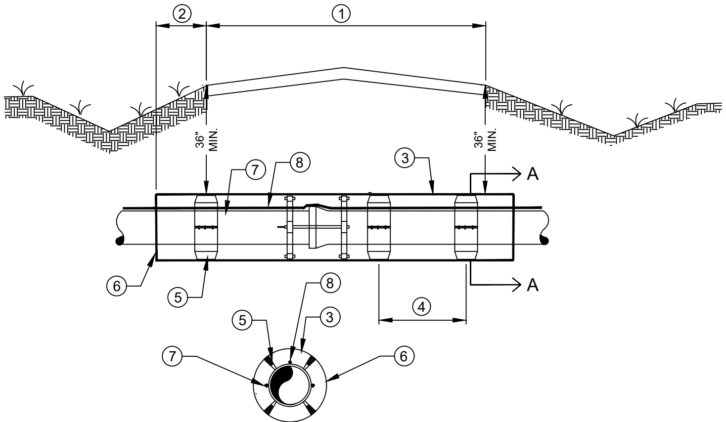
SECTION A-A
